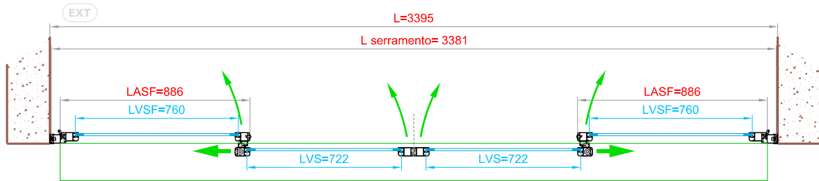
sezione orizzontale ANTA CHIUSA
