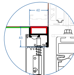
sezione verticale
