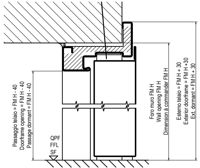
Sezione verticale Vertical cross section Coupe vertical
