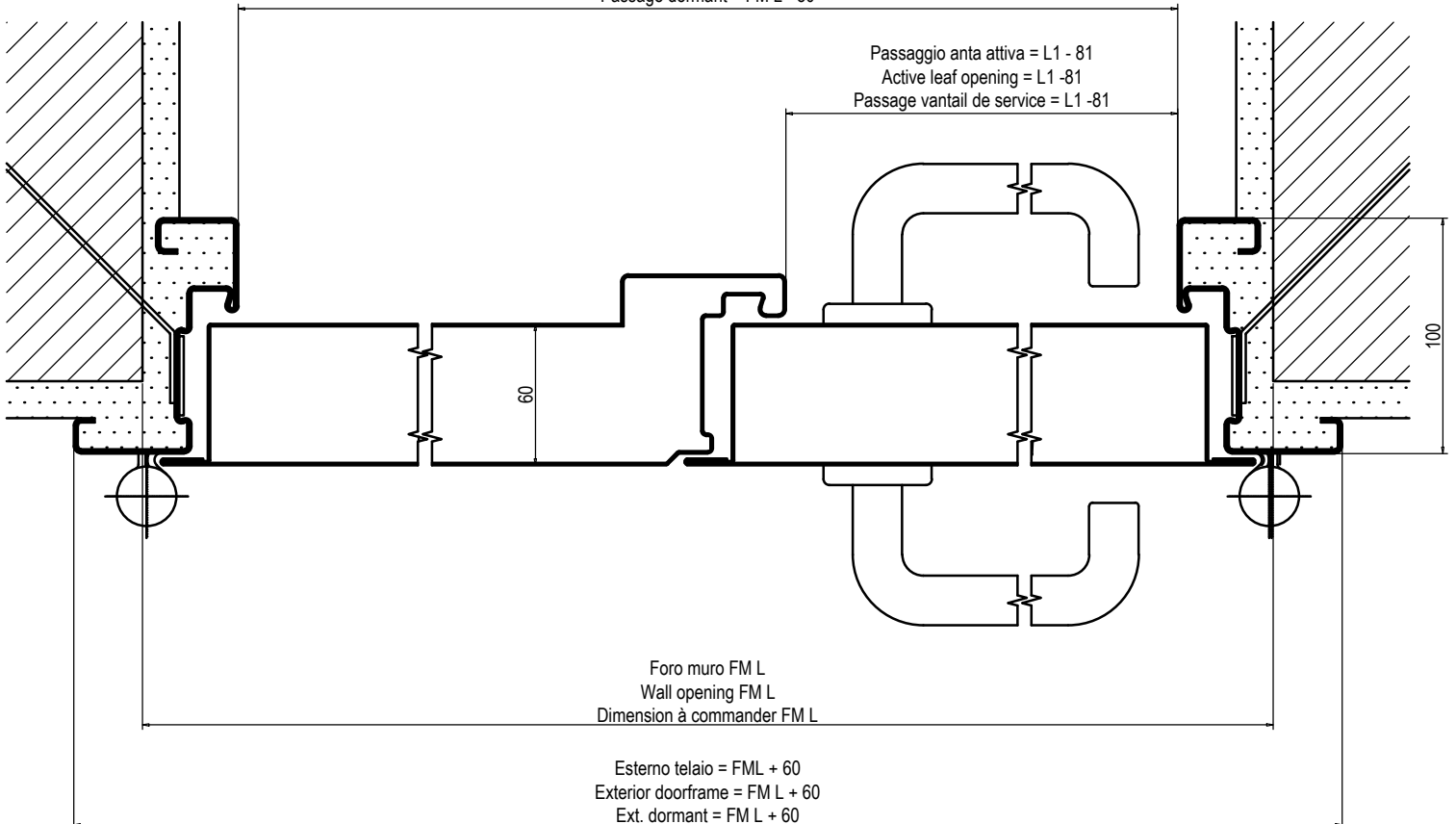
Sezione orizzontale Horizontal cross section Coupe horizontale
